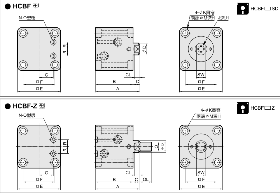
外形尺寸表
