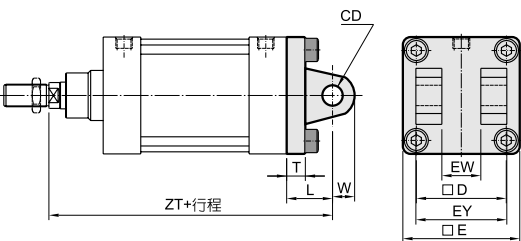
外形尺寸表
