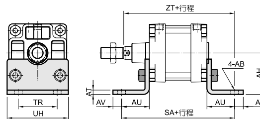
外形尺寸表
