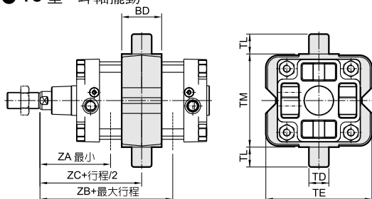
外形尺寸表
