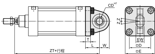
外形尺寸表
