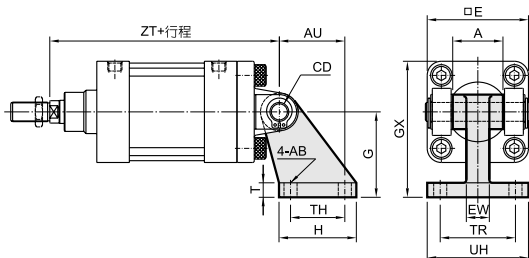
外形尺寸表
