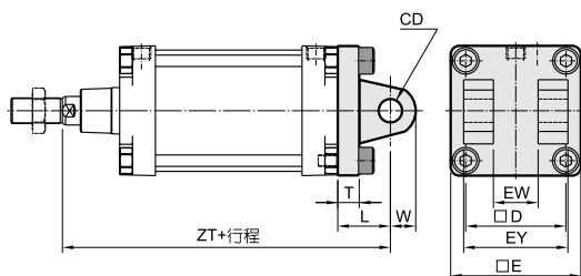
外形尺寸表
