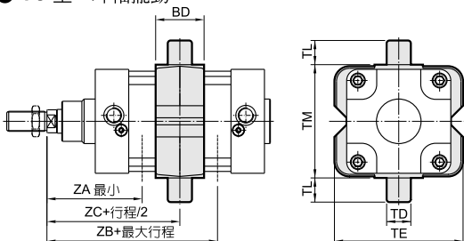
外形尺寸表
