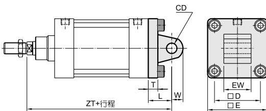
外形尺寸表
