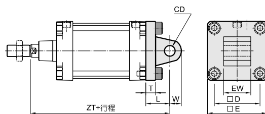
外形尺寸表
