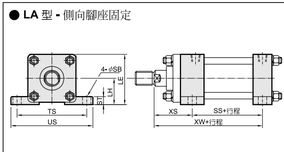
外形尺寸表
