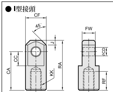
外形尺寸表
