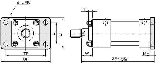
外形尺寸表
