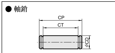
外形尺寸表
