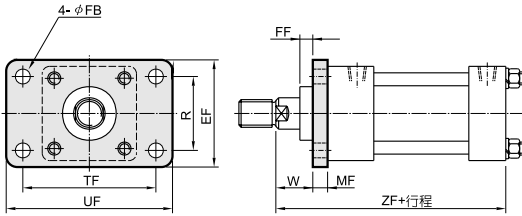
外形尺寸表
