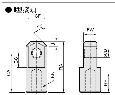
外形尺寸表
