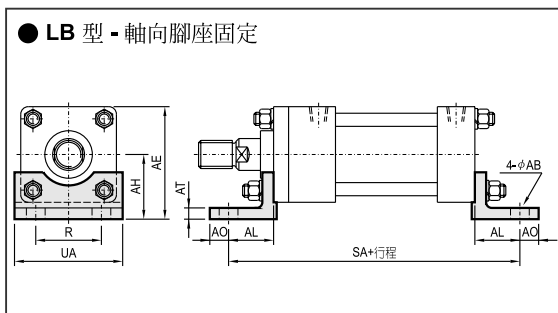
外形尺寸表
