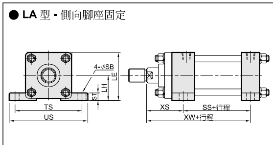
外形尺寸表
