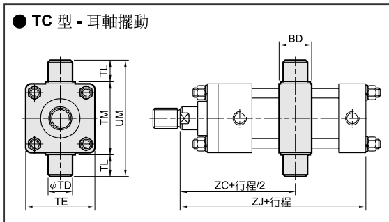
外形尺寸表
